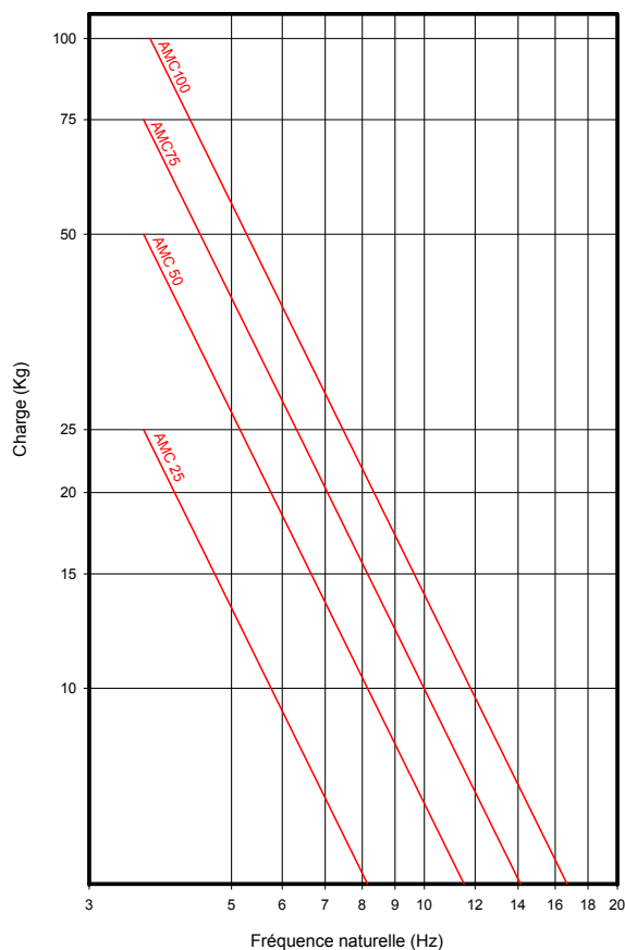
FREQUENCE PROPRE
